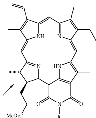
Chlorin (purpurinimide)
